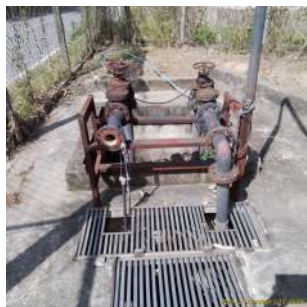
Foto 1 - Poço de sucção com uma bomba.
