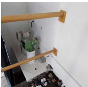
Foto 5 - Dosadoras químicas na elevatória nova.
