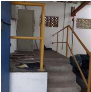
Foto 1 - Guarda-corpo da elevatória nova.
