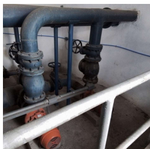
Foto 3 - Vista do booster da ETA Cerejeiras do Saae Atibaia.
