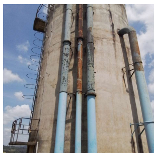
Foto 1 - Guarda-corpo fora dos padrões adequados do Reservatório elevado da ETA Cerejeiras do Saae Atibaia.
