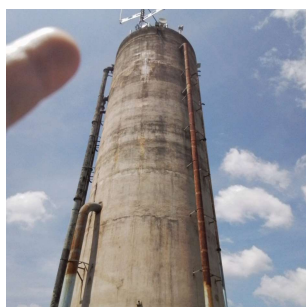
Foto 1 - Vista do Reservatório elevado da ETA Cerejeiras do Saae Atibaia.
