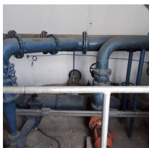
Foto 1 - Vista do booster da ETA Cerejeiras do Saae Atibaia.
