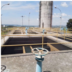
Foto 6 - Vista da ETA Cerejeiras do Saae Atibaia.
