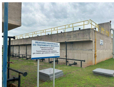
Foto 12 - Reatores UASB
