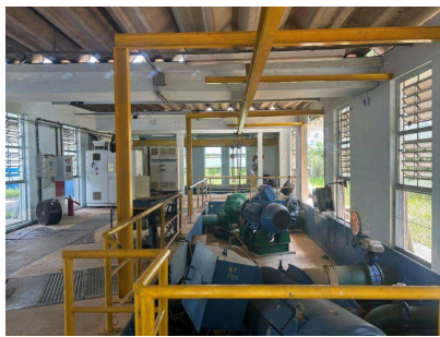
Foto 5 - Conjuntos moto-bomba
