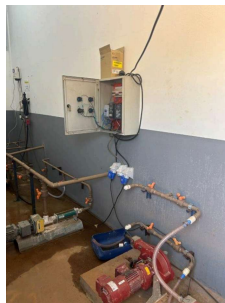
Foto 18 - Bombas dosadoras
