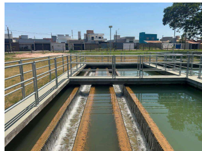
Foto 16 - Decantação
