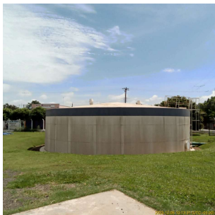
Foto 1 - Reservatório apoiado Santa Fé (R400)
