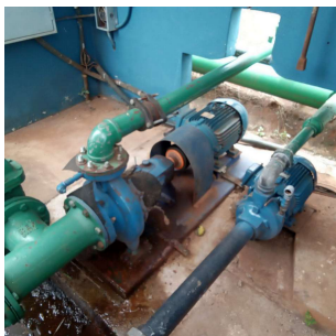
Foto 5 - Recalque para Reservatório elevado Santa Fé
