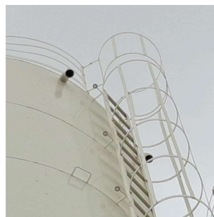
Foto 2 - Ausência de tela de proteção no tubo extravasor.
