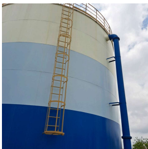
Foto 8 - Guarda-corpo da escada marinheiro e tubulação de chegada de água vinda do res. pulmão.
