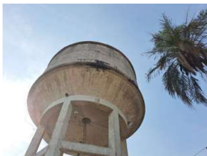
Foto 1 - Marcas de vazamentos na lateral do reservatório.
