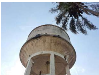
Foto 3 - Marcas de vazamentos na lateral do reservatório.
