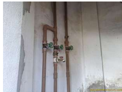
Foto 2 - Tubulações de subida e descida dentro da base do reservatório, com destaque para torneira de tomada de água bruta.
