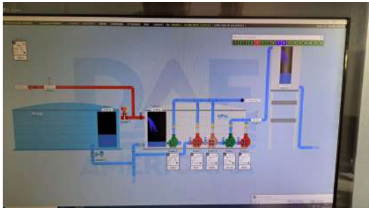
Foto 1 - Sistema de telemetria do Centro de Reservação Chácara Letônia.
