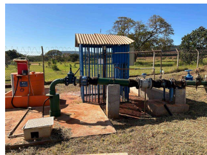
Foto 4 - Barrilete do poço
