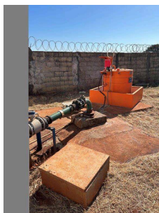
Foto 3 - Macromedidor e tanque de flúor
