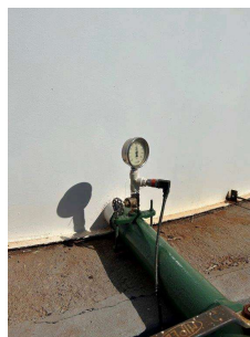
Foto 4 - medição de nível - manômetro
