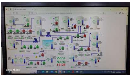
Foto 1 - Sistema de telemetria do abastecimento de água de Mogi Guaçu.
