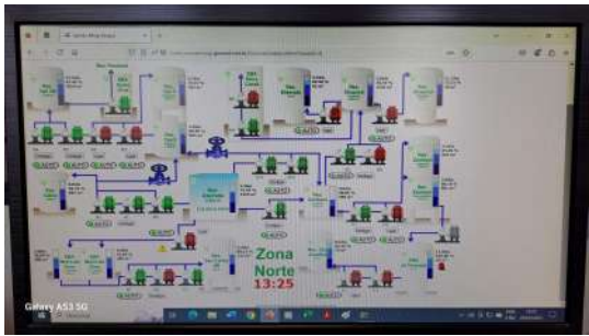
Foto 1 - Telemetria do sistema de abastecimento de água de Mogi Guaçu.
