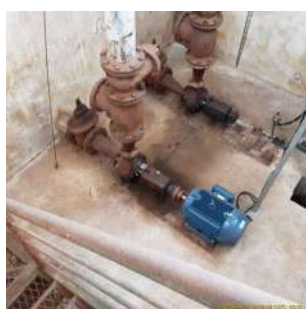
Foto 1 - Vista interna da estação elevatória de esgoto Eco Tecnológico Damha
