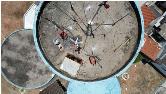
Foto 1 - Tampa do reservatório elevado apresenta pontos de corrosão.
