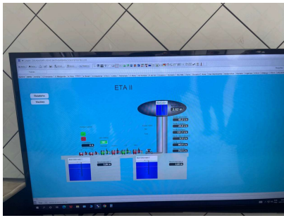
Foto 1 - Telemetria na ETA 2 em Santa Bárbara DOeste
