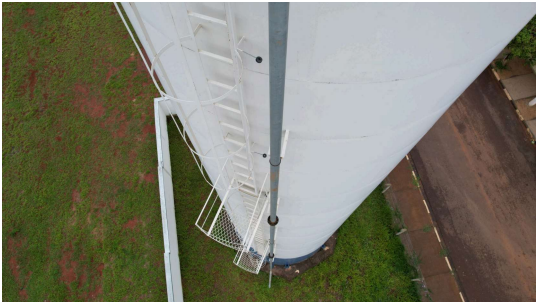
Foto 2 - Reservatório Vila Salemi - vista lateral e ausência de cabo de aterramento na estrutura de descida.
