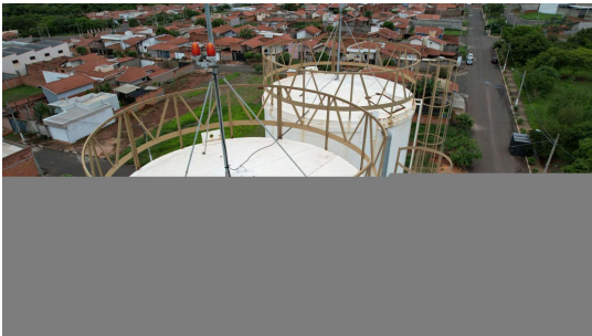
Foto 4 - Reservatório Santa Carolina visto de cima com foco em tampas
