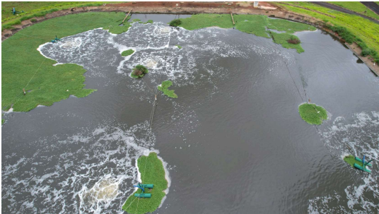
Foto 2 - ETE Tambau - lagoa aerada
