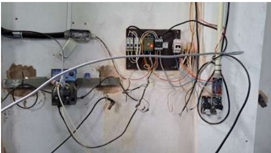
Foto 2 - Situação da instalação elétrica das bombas dosadoras instaladas na base do Reservatório Ubá 1
