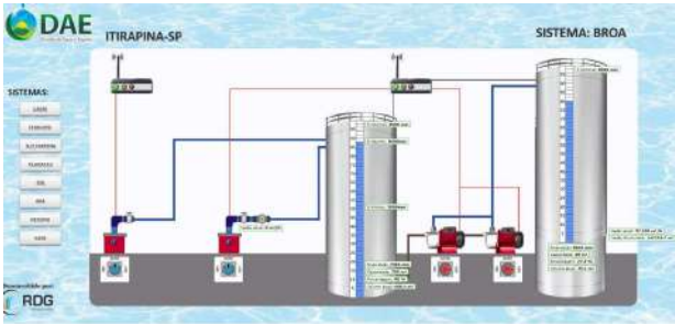
Foto 1 - Telemetria - Sistema Broa
