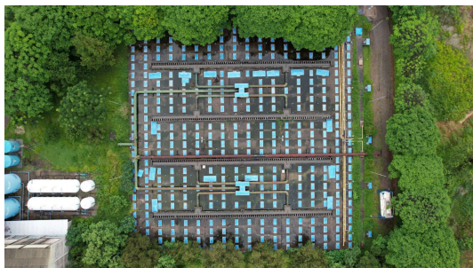
Foto 2 - ETE Capuava vista por cima com enfoque nos reatores anaeróbios (UASB)
