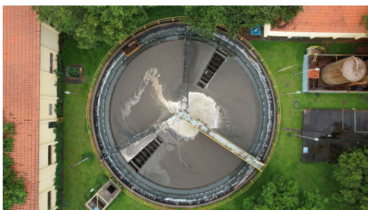
Foto 3 - Flotador da ETE Capuava visto por cima
