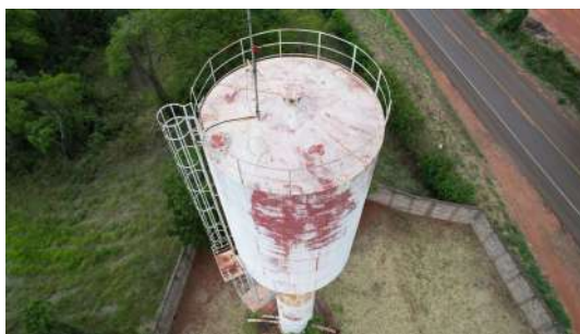
Foto 2 - Imagens captadas com auxílio de drone no dia 28/11/2022 da tampa de inspeção do Reservatório Portal das Laranjeiras em Araraquara
