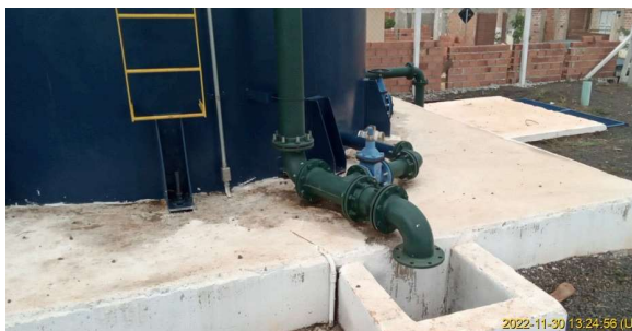
Foto 3 - Vista do sistema de extravasamento.
