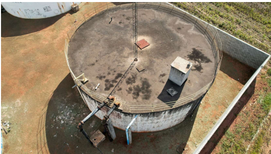
Foto 2 - Vista superior do reservatório Klavin 1
