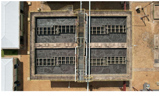
Foto 3 - Vista superior dos reatores UBOX
