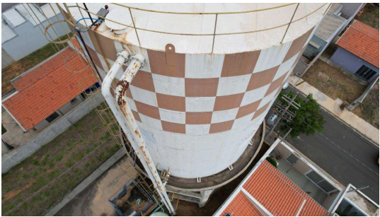
Foto 6 - Parte superior lateral do Reservatório R22 - Sistema Terra Nova com detalhe de extravasor
