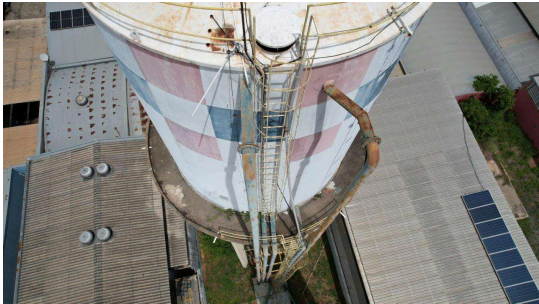
Foto 1 - Detalhe de tampa de inspeção parcialmente aberta
