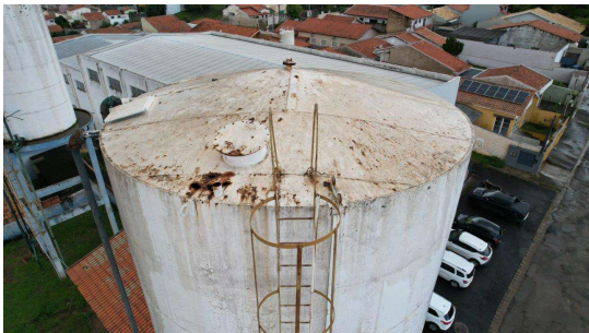
Foto 1 - Parte superior do Reservatório R7 - Sistema Cohab com furos e corrosão em estado avançado
