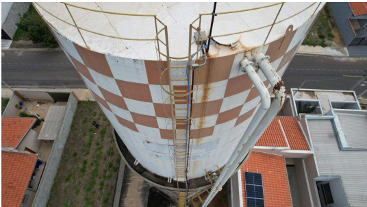
Foto 4 - Parte lateral do Reservatório R22 - Sistema Terra Nova com detalhe de escada com guarda-corpos
