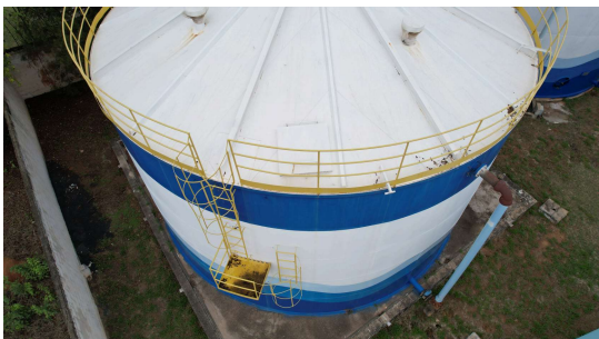
Foto 3 - Acesso a reservatório, telas contra entrada de inseto e tampa de inspeção regulares
