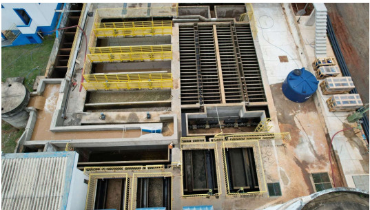
Foto 4 - Unidades de tratamento da ETA Vila Progresso
