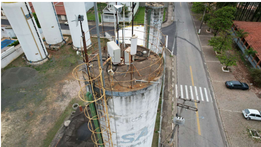
Foto 3 - Detalhe de descida do para-raios - CR BEPIM
