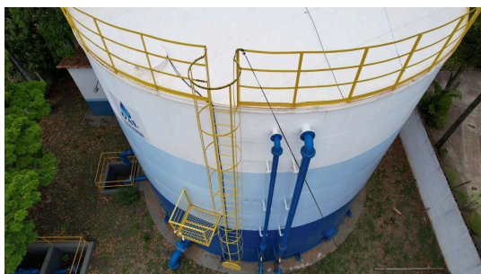
Foto 1 - Vista geral do Reservatório apoiado BROA
