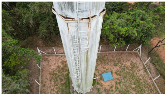
Foto 4 - Regiões com marcas de oxidação no Reservatório Uba 2
