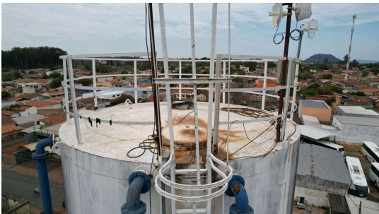
Foto 5 - Oxidação na tampa de inspeção - Reservatório elevado Rua Cinco
