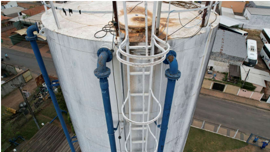
Foto 4 - Oxidação na tampa de inspeção - Reservatório elevado Rua Cinco
