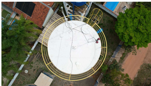
Foto 2 - Vista geral - Reservatório elevado BROA
