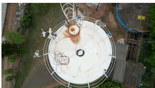
Foto 1 - Oxidação na tampa de inspeção e em seu entorno - Reservatório elevado Rua Cinco
