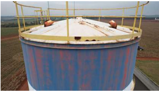
Foto 1 - Tubulações de ventilação do Reservatório elevado Jardim Empyrio em Leme
