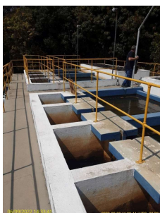
Foto 11 - Decantadores da ETA Monte Alegre
