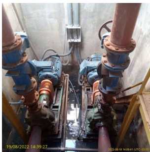
Foto 1 - Existência de vazamentos nas bombas da EEE Zona Norte
