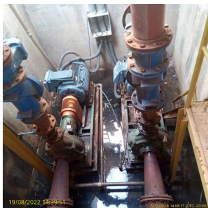
Foto 1 - Vista do interior da elevatória
