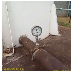
Foto 4 - Manômetro do Reservatório Residencial Lagoa
