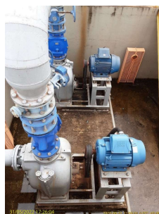
Foto 10 - Detalhe das bombas.
