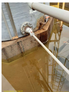
Foto 1 - Vazamento aparente (gotejamento) no tanque de cloro.
