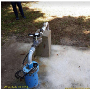
Foto 1 - Detalhe do poço sem torneira para coleta de água
