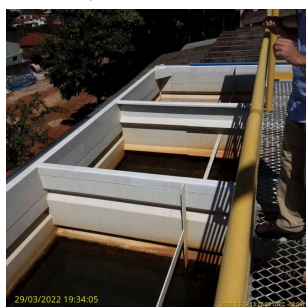
Foto 9 - Vista geral do alto da ETA Compacta
