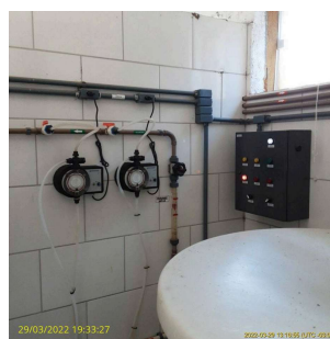
Foto 2 - Detalhe das bombas dosadoras
