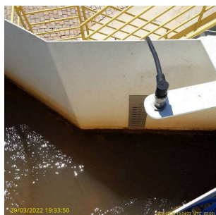
Foto 7 - Chegada da água bruta e medição da vazão pela Calha Parshall
