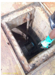
Foto 1 - Gradeamento no poço de sucção da elevatória de esgoto.
