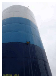
Foto 2 - Tubo sem tela de proteção; medidor de nível do reservatório.
