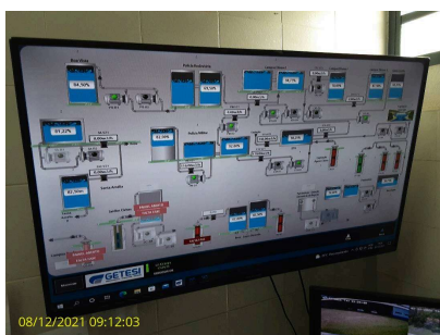
Foto 1 - Sistema de telemetria em funcionamento.
