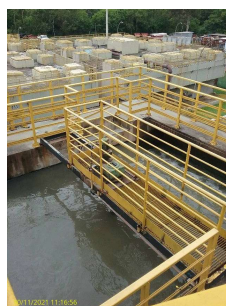
Foto 6 - Desarenador
