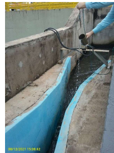
Foto 22 - Calha Parshall Saída
