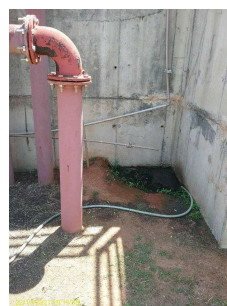
Foto 2 - Drenagem inadequada de esgoto próximo a caixa de distribuição para os decantadores
