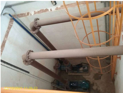
Foto 4 - Sem bomba reserva
