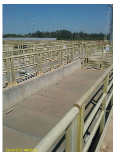
Foto 8 - Tratamento preliminar - caixa de areia
