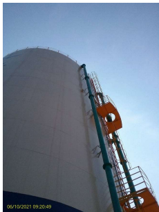
Foto 1 - Escada de acesso à cobertura e guarda-corpo
