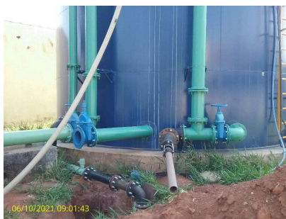
Foto 3 - Descarga de fundo
