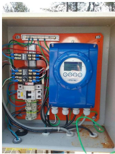
Foto 1 - Macromedidor de entrada
