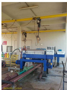
Foto 1 - Centrífugas para tratamento do lodo
