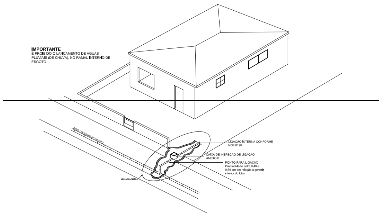
Figura 01: Exemplo de instalação de ramal predial de esgoto residencial.
