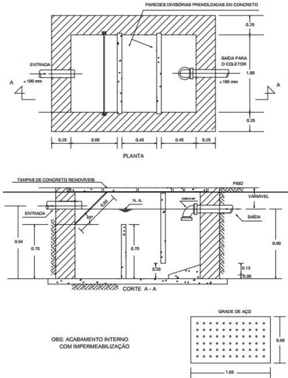
Figura 07: Caixa retentora de resíduos de fabricação de pisos (ardósia, granito, mármore, etc.).
