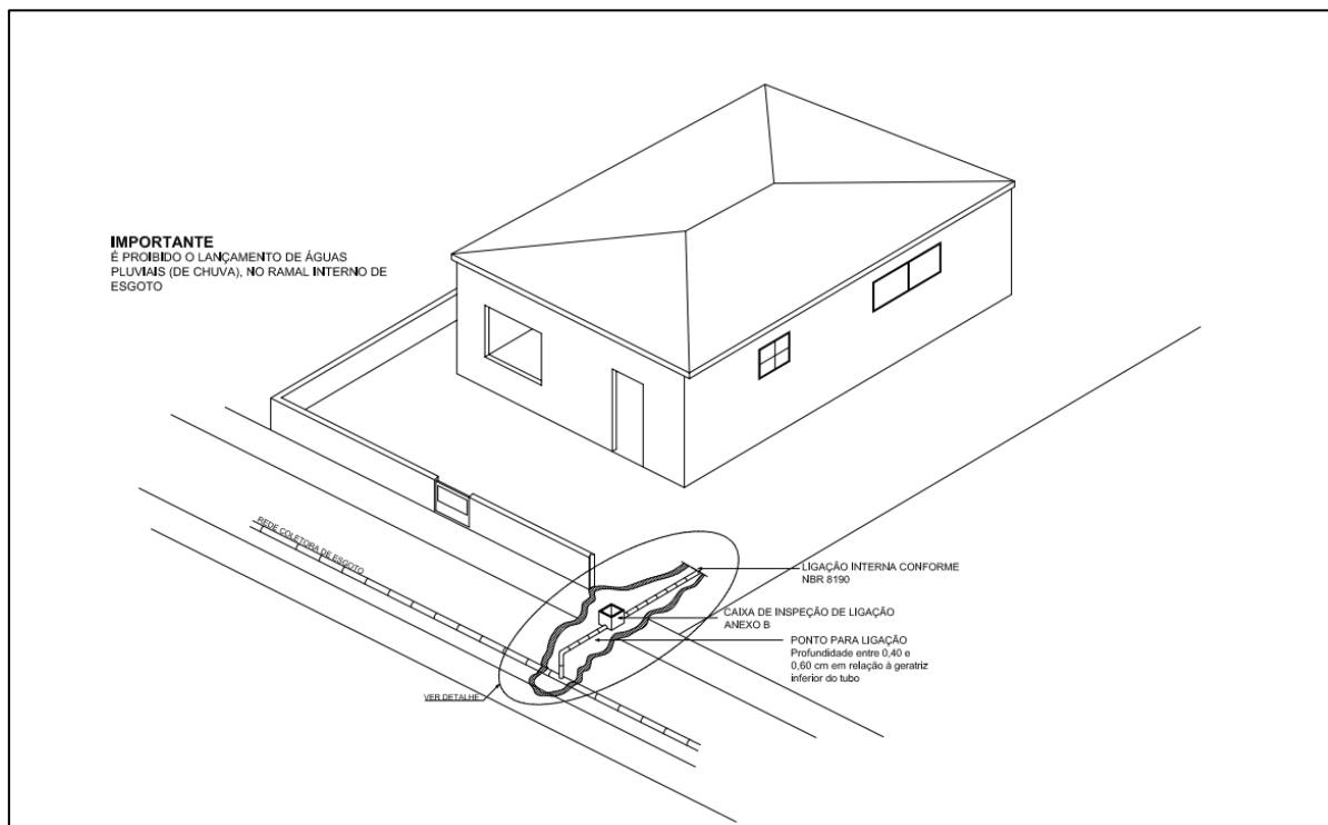
Figura 01: Exemplo de instalação de ramal predial de esgoto residencial.
