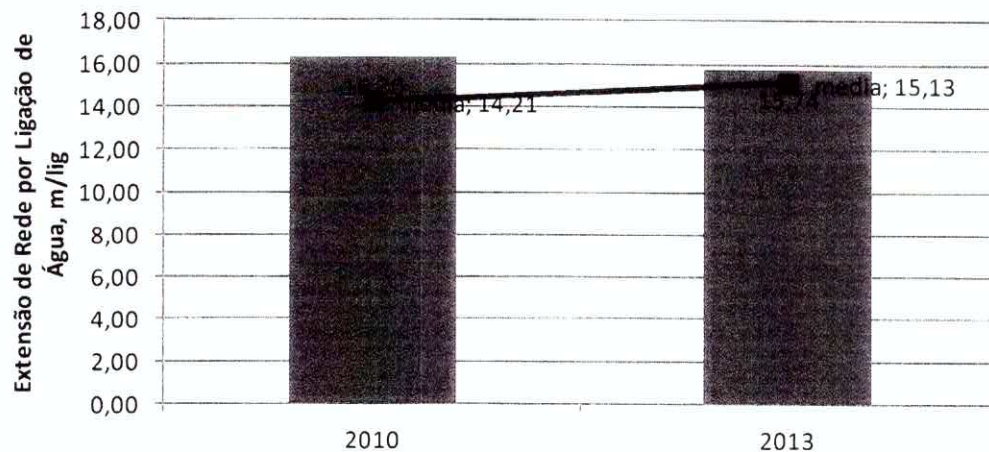
Figura 5: Extensão de rede de água por ligação (m/ligação)
