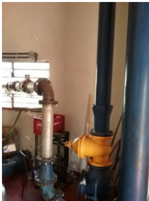
Descrição(4): Tubulações do barrilete de recalque, embaixo do Reservatório Elevado
