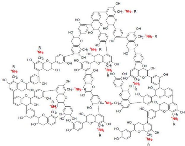
Estrutura do tanino
