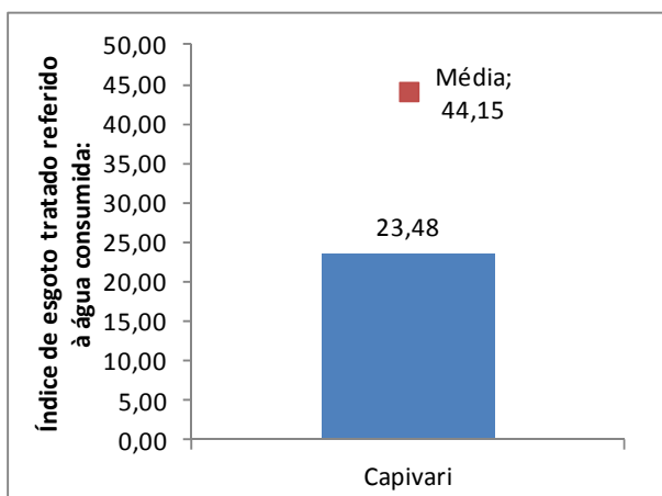
Figura 27 - Índice de tratamento de esgoto em relação à água consumida (SNIS 2013)
