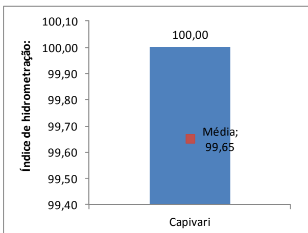
Figura 23 - Índice de micromedição (SNIS 2013)
